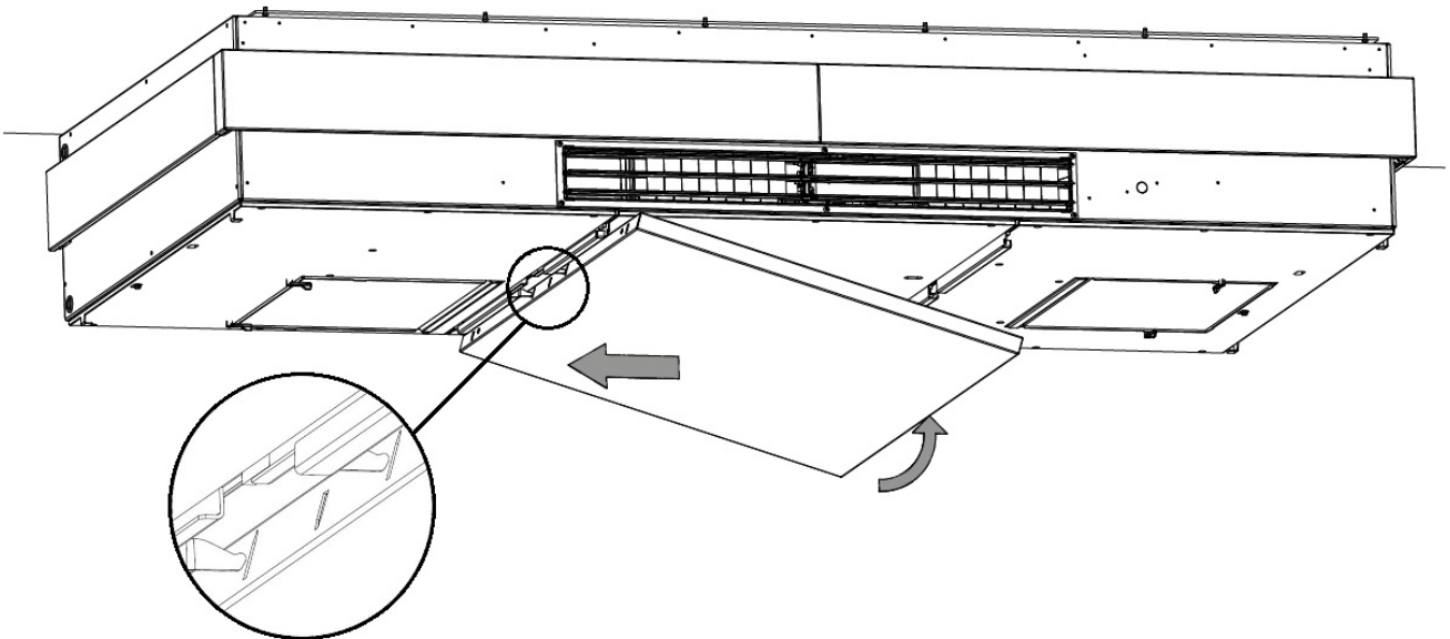
Abbildung 51: Aufsetzen des mittleren Gehäusedeckels auf die Scharniere
