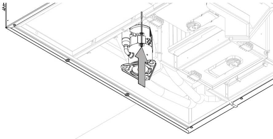
Abbildung 22: Transportsicherung
