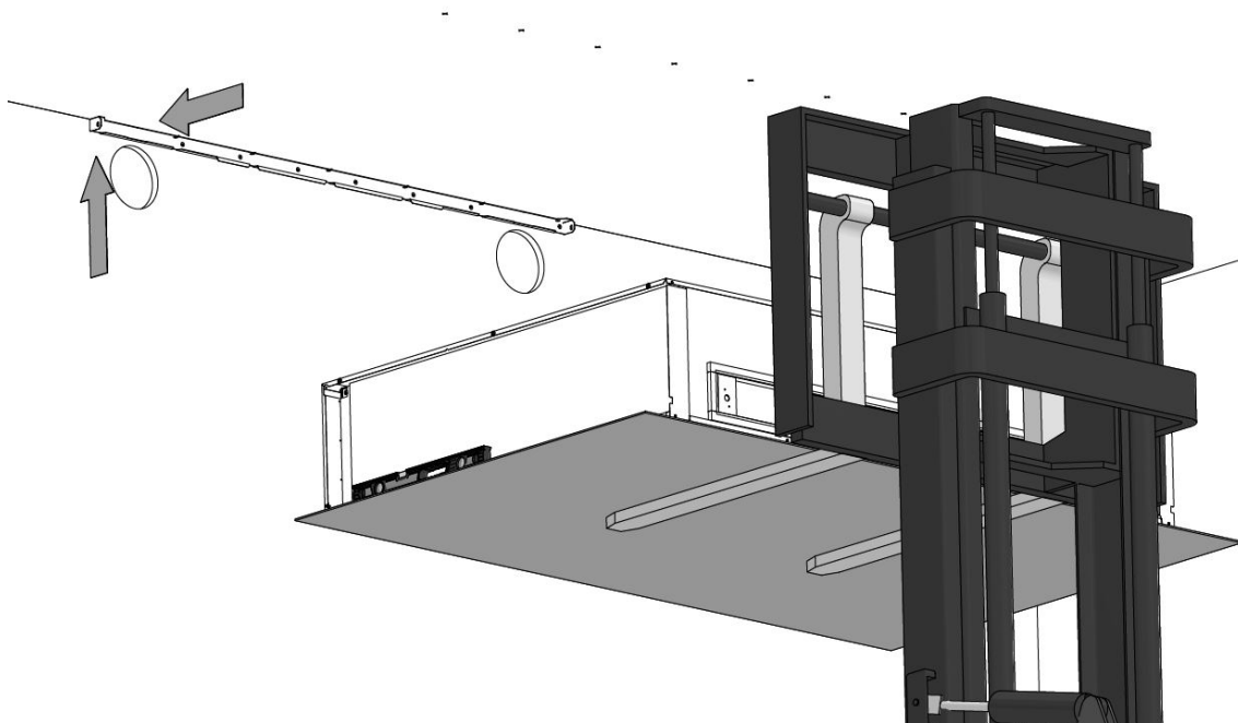
Abbildung 18: Heben Sie das Gerät hoch und setzen Sie es auf die Halterung
