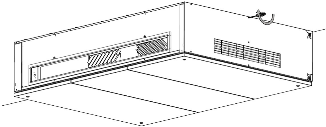
Abbildung 23: Montieren Sie die rechte Seitenabdeckung wieder
