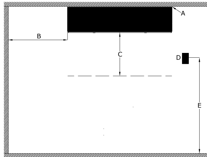
Abbildung 5: Mindestabstand zu Gebäudeteilen, AM 950 C-Gerät
