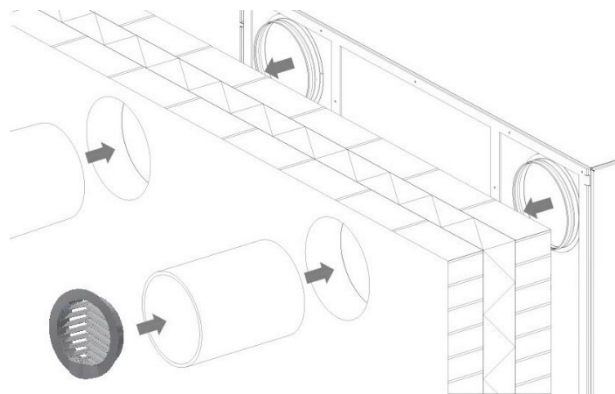
Abbildung 29: Kanalrohre und Gitter – allgemeiner Überblick
