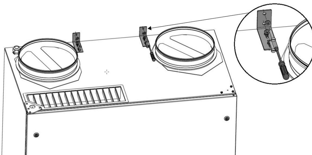
Abbildung 28: Befestigen Sie die Halterungen an der Geräteoberseite an der Wand
