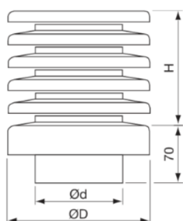
Außenlufthaube
