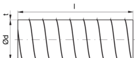
3m Lüftungskanal
