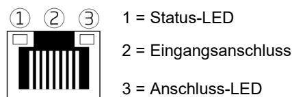
Abbildung 28: Ethernet, RJ45
