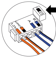
Abbildung 25: DIP-Schalter geschlossen („ON“)
