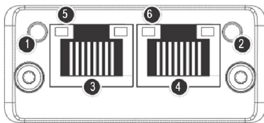
Abbildung 33: BACnet™ /IP
