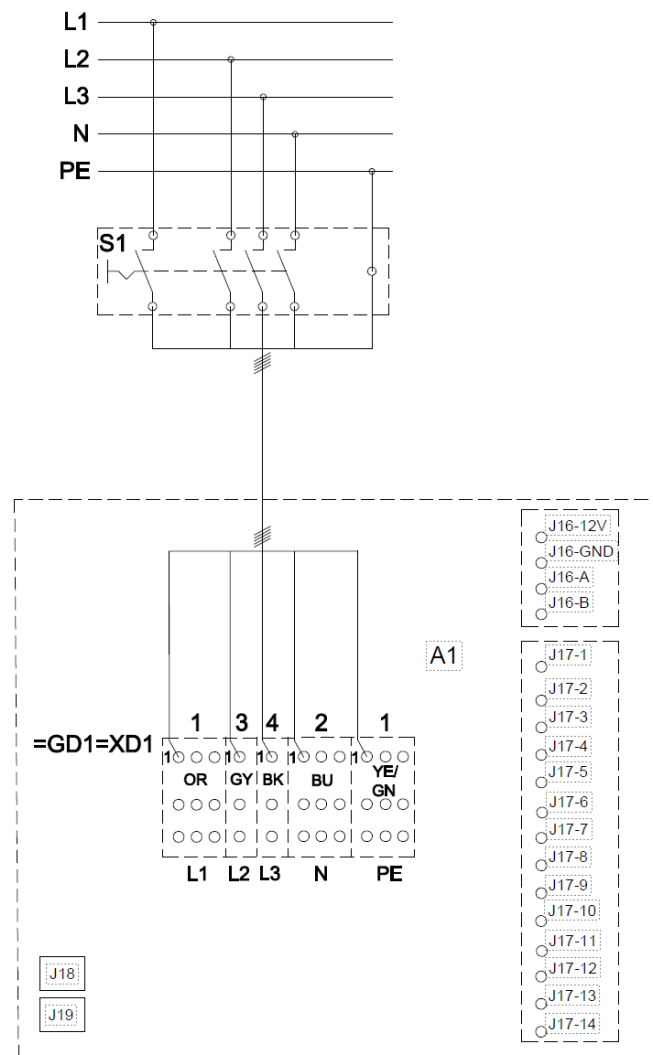
Abbildung 8: Steuerbox, Standardkonfiguration
