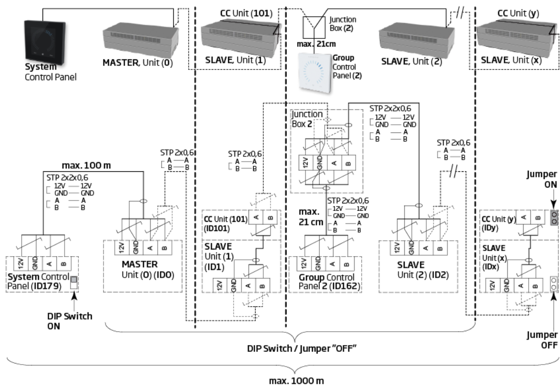
Abbildung 24: Airlinq-BMS-Installation Übersicht
