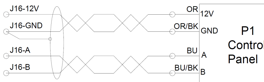
Abbildung 19: Installation des Bedienpaneels, Steuerbox und Paneel
