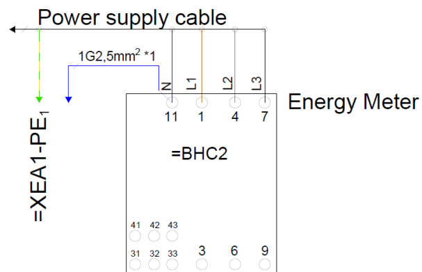
Abbildung 16: Energiezähler, 3-Phase
