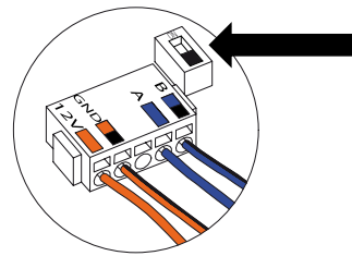
Abbildung 26: DIP-Schalter offen („OFF“)
