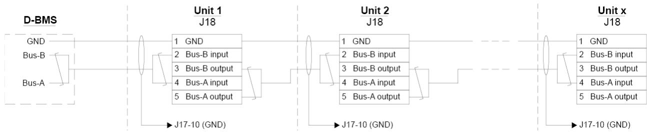
Abbildung 32: MODBUS®, Geräteanschlüsse
