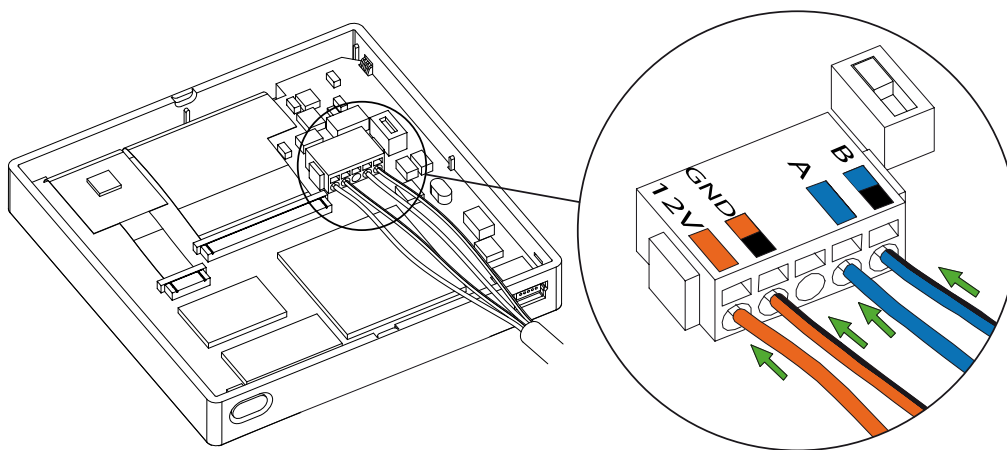
Abbildung 20: Installation des Bedienpaneels, Airlinq® Orbit-Paneel
