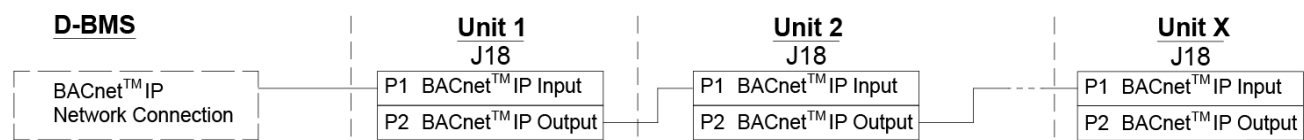
Abbildung 35: BACnet™ /IP, Geräteanschlüsse
