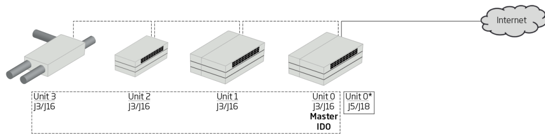
Abbildung 31: Airlinq BMS und Airlinq® Online, Geräteanschlüsse
