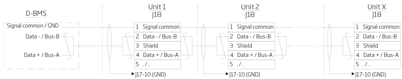
Abbildung 37: BACnet™ MS/TP, Geräteanschlüsse
