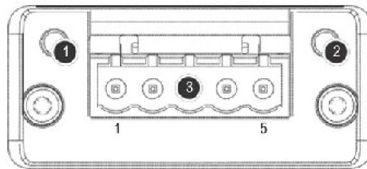
Abbildung 36: BACnet™ MS/TP
