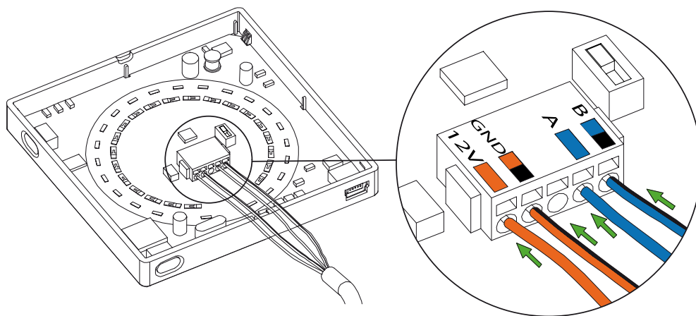
Abbildung 23: Installation des Bedienpaneels, Airlinq® Viva-Paneel
