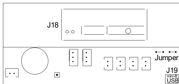
Abbildung 10: BMS/Ethernet (J18), PC-Kommunikation (J19), Steckbrückeneinstellung
