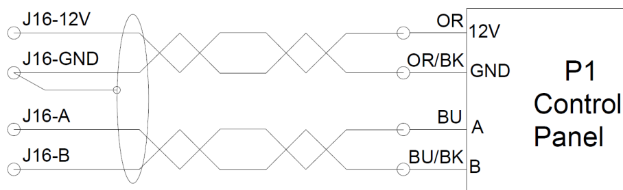
Abbildung 22: Installation des Bedienpaneels, Steuerbox und Paneel
