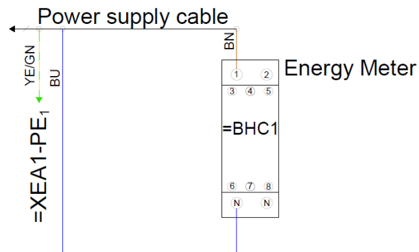
Abbildung 15: Energiezähler, 1-Phase
