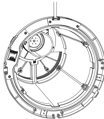
Abbildung 5 - Wandbefestigung und äußere Teil
