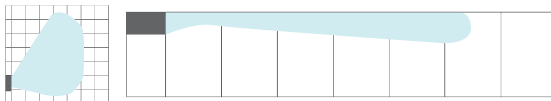
Asymmetrische Abstrahlung, wahlweise nach links oder rechts
