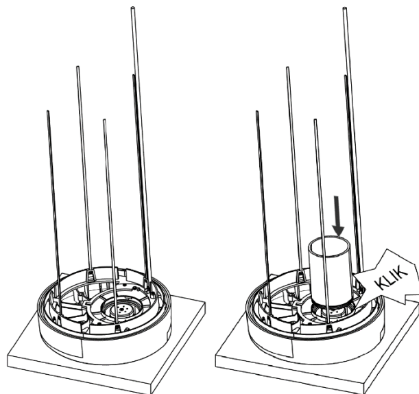
Abbildung 10 - Vorbereitung der Außenkappe mit Ø90-mm-Rohr
