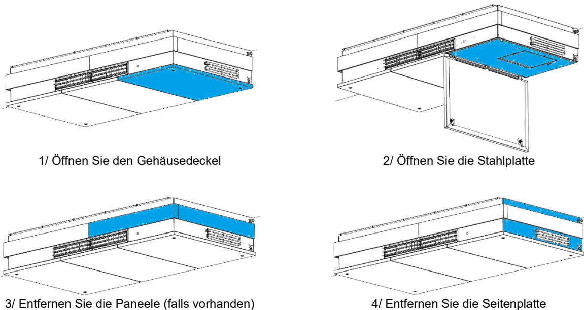
Abbildung 3: Zugang zu Anschlüssen erhalten
